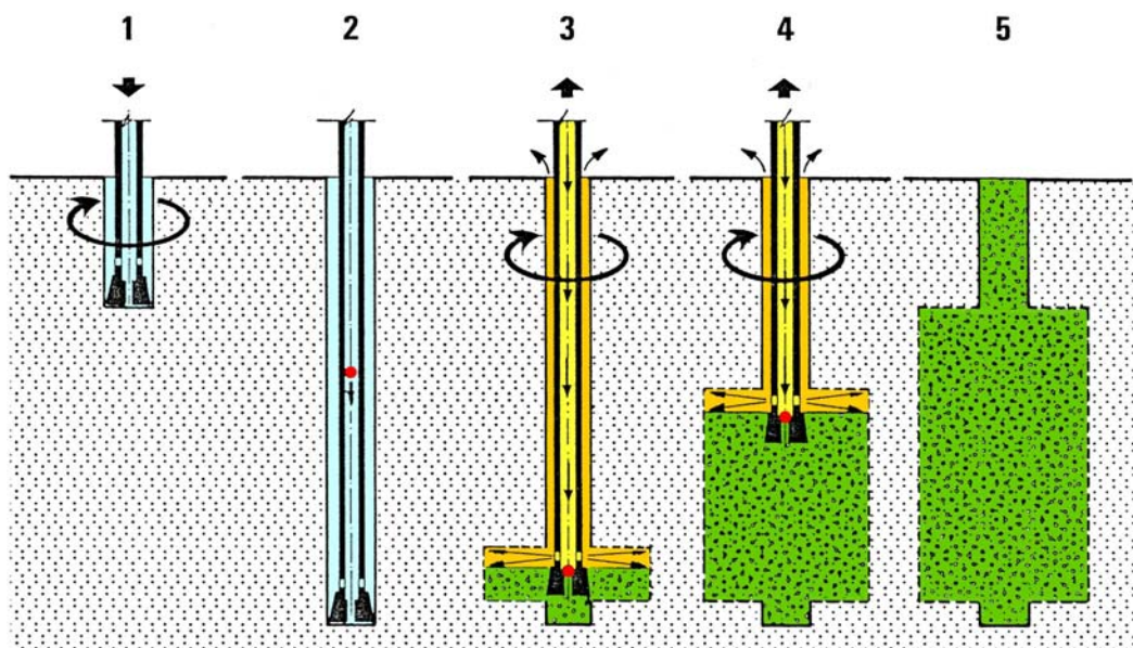
Fig. 1. Secuencia de operaciones del Jet-Grouting
